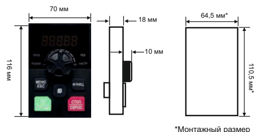
Монтажная рамка
