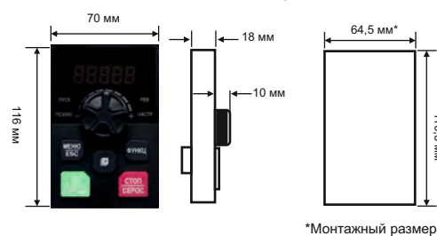
Монтажная рамка
